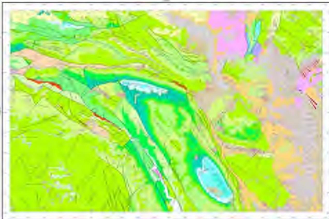
Mapa Geològic d'Espanya, full 746/28-29 (Llombai). Font: IGME
