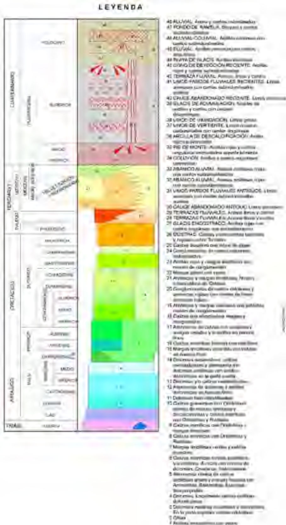
Llegenda per al mapa Geològic d'Espanya, full 746/28-29 (Llombai). Font: IGME
