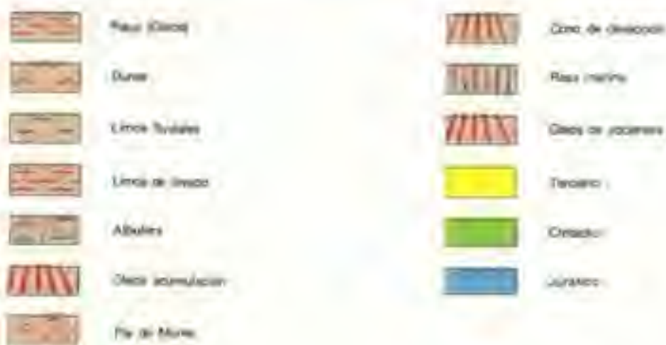
Esquema tectònica geomorfològic. Font: IGME
